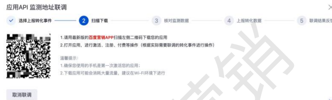
图 4.联调扫码
